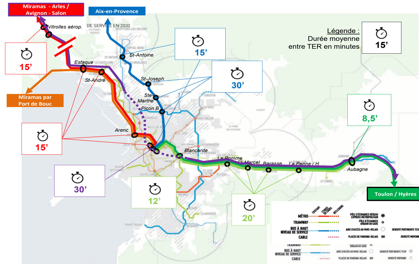
Figure 25 : Vers un RER métropolitain - schéma des dessertes et des fréquences à l'échelle de Marseille
