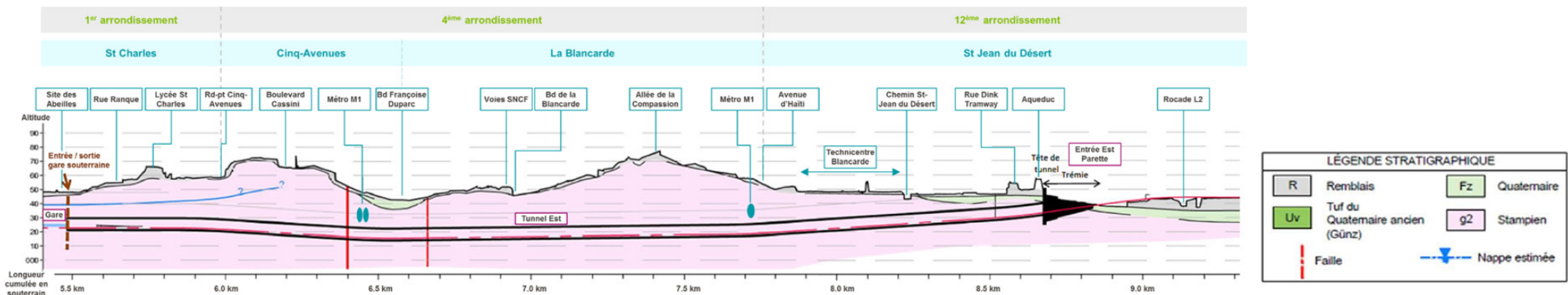
Figure 68 : Profil en long du tunnel de Marseille
