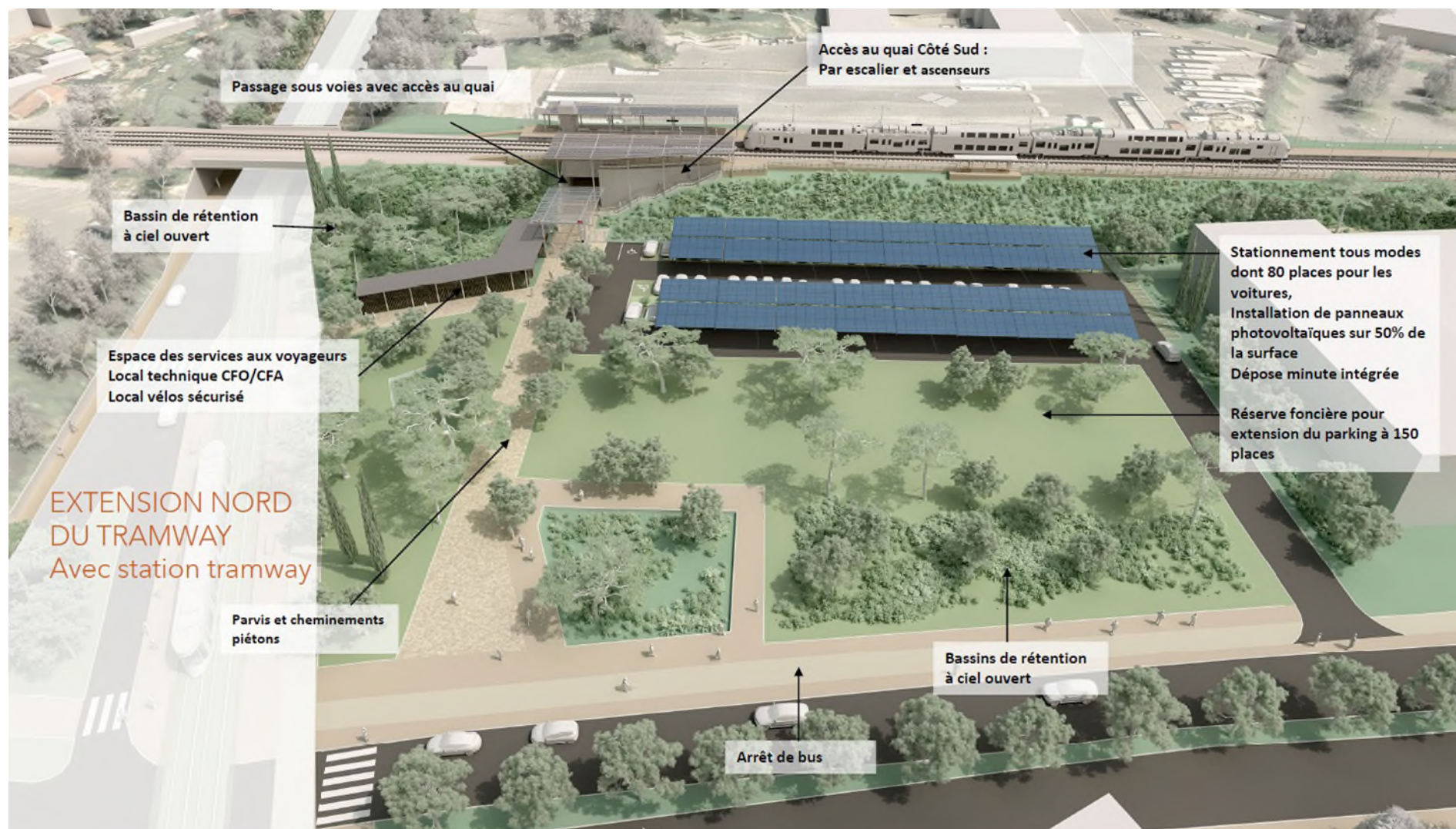
Figure 57 : Aperçu de la future halte de Saint-André – AREP 2024
