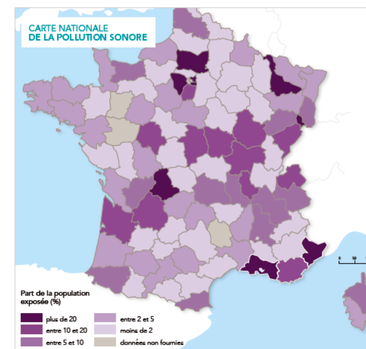
Figure 15 : Pollution sonore au niveau national (SNCF-R, 2016)
