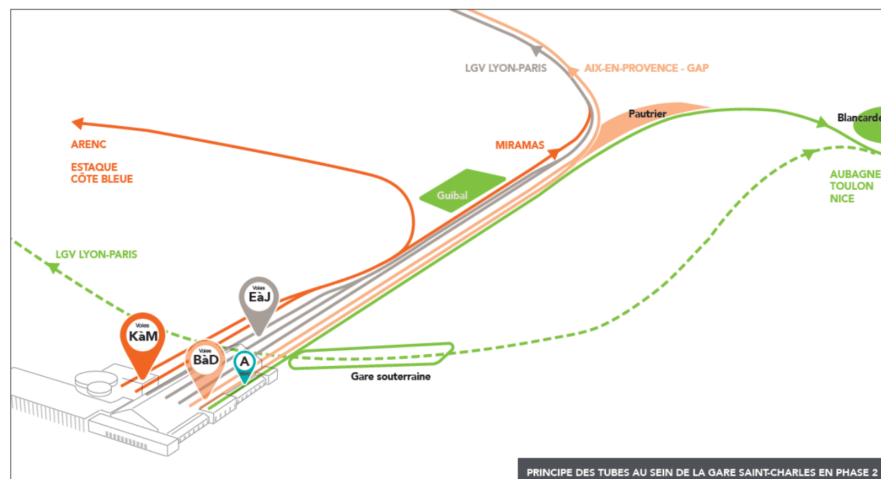
Figure 50 : Principe de réorganisation du plateau Saint-Charles
