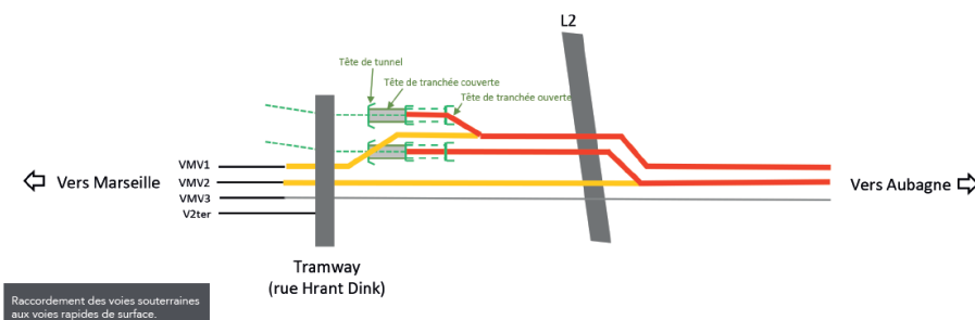
Figure 73 : Principe de raccordement des voies du tunnel avec les voies rapides provenant du plateau de surface
