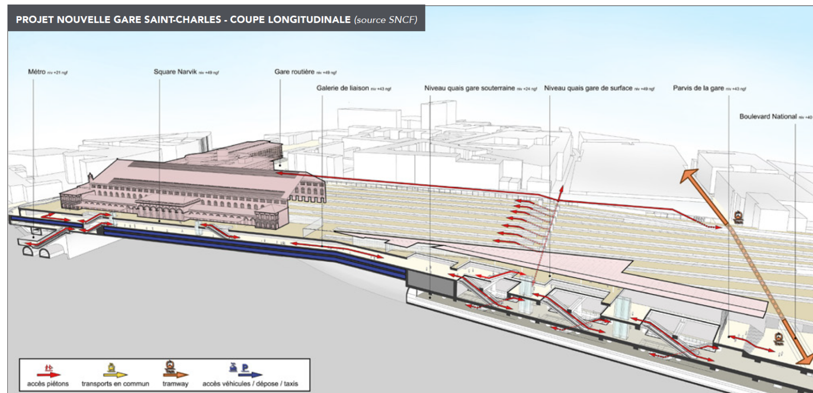
Figure 65 : Coupe longitudinale montrant les principaux cheminements
