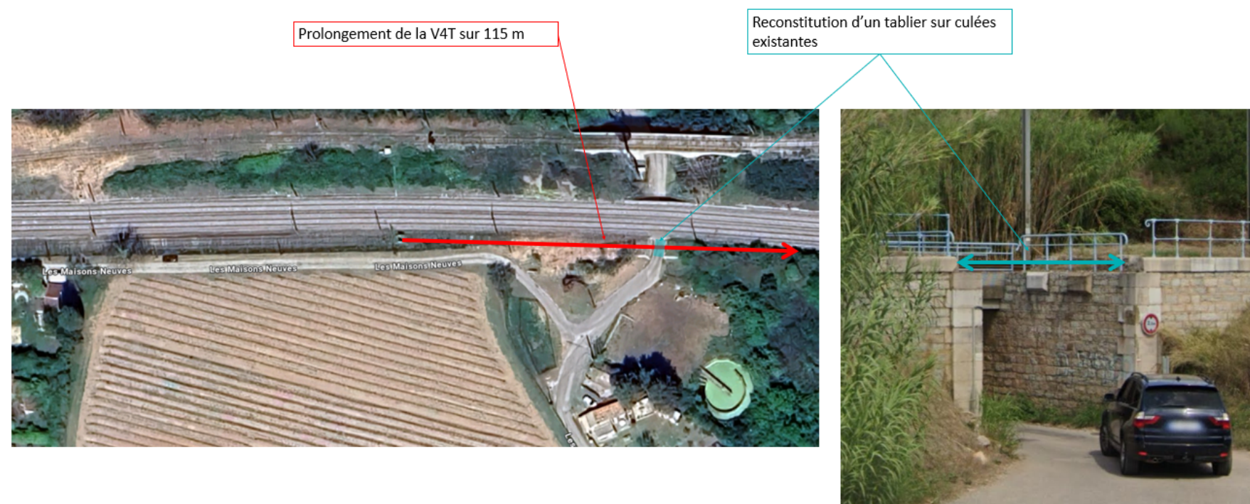
Figure 45 : localisation du prolongement de la V4T et des travaux sur le pont-rail du chemin des Maisons-Neuves (Egis, AVP – 2024)
