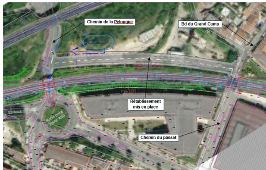
Figure 58. Tracé du rétablissement routier (Source : SETEC)
