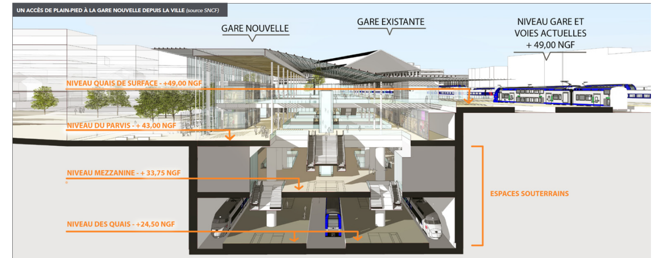
Figure 67 : Vue en coupe de la nouvelle gare souterraine
