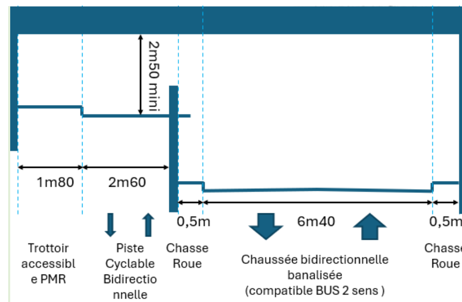
Figure 61 : Coupe en travers du pont rail Cauvet (Source : SETEC)
