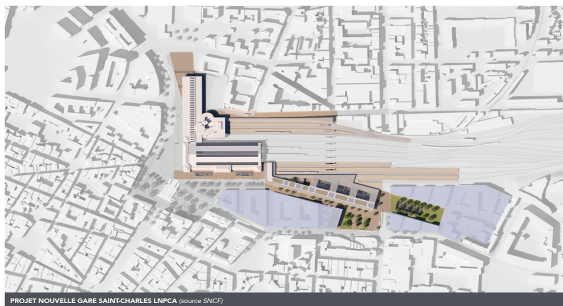
Figure 64 : Plan général de la future gare souterraine, avec les éléments de surface de la gare souterraine
